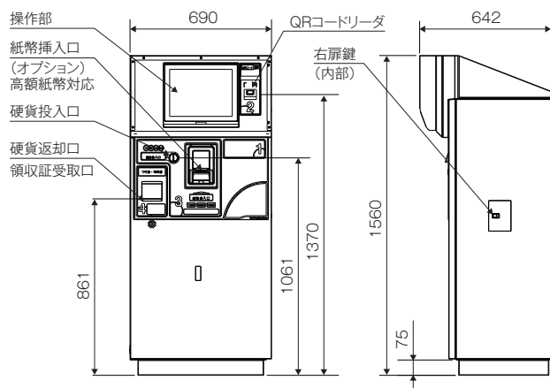
FGL-200 事前精算機
