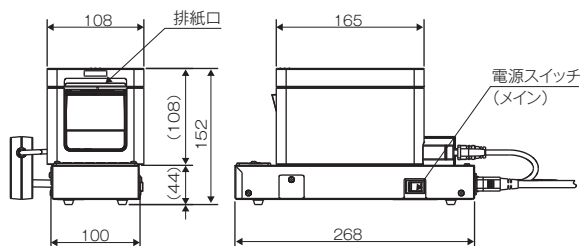
TE-200/QR QRコードサービス券発券機
